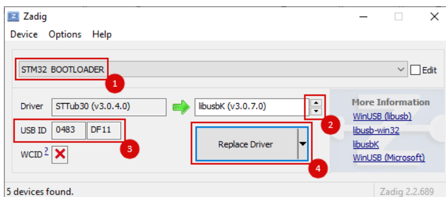
Рисунок А.2 – Окно программы «Zadig»
