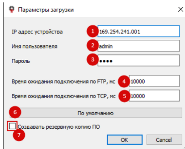
Рисунок А.16 – Окно параметров загрузки
