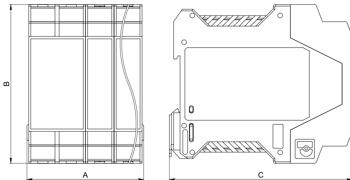
Рисунок 1.5 – Габаритные размеры устройства
