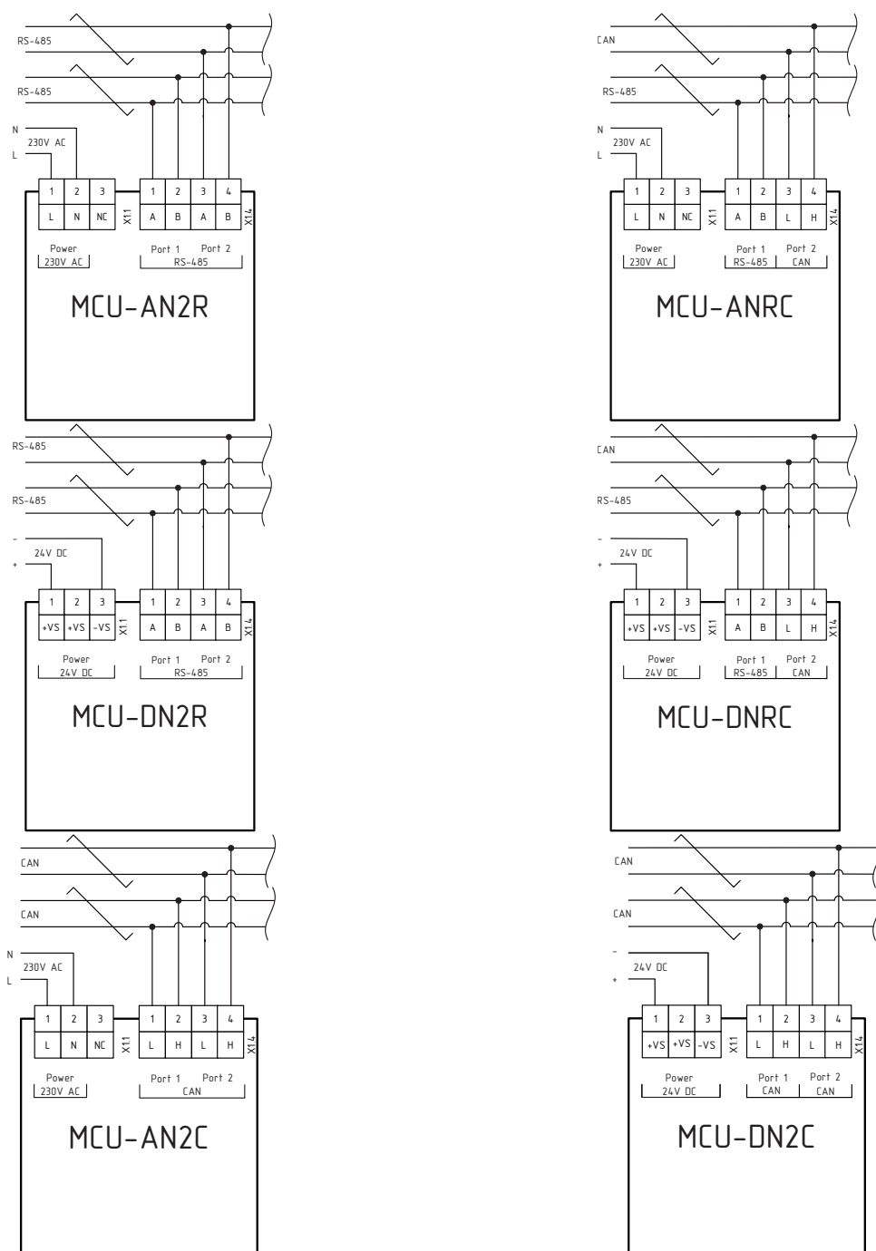
Рисунок 1.6 – Схемы подключения
