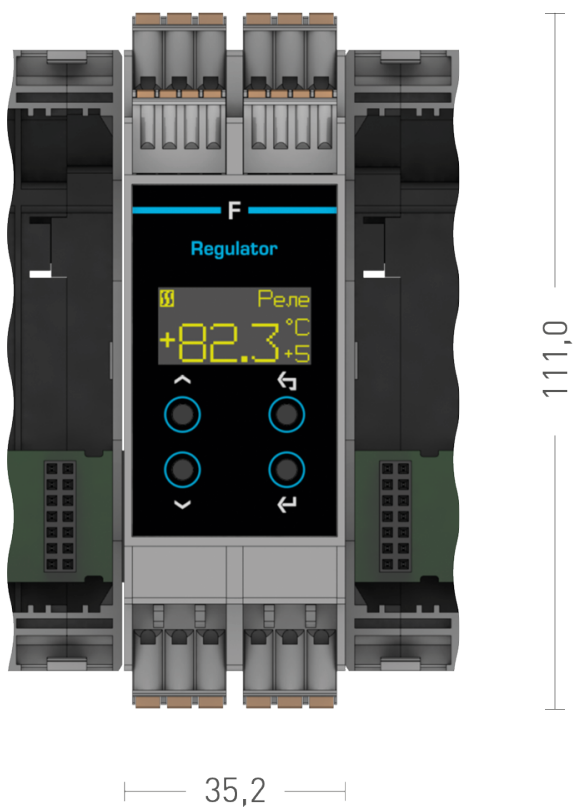
Рисунок 1.18 – Внешний вид модуля расширения MCU-F
