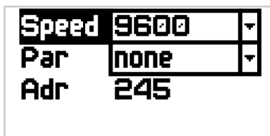
Рисунок E.14 – Настройки протокола связи по протоколу RS-485
