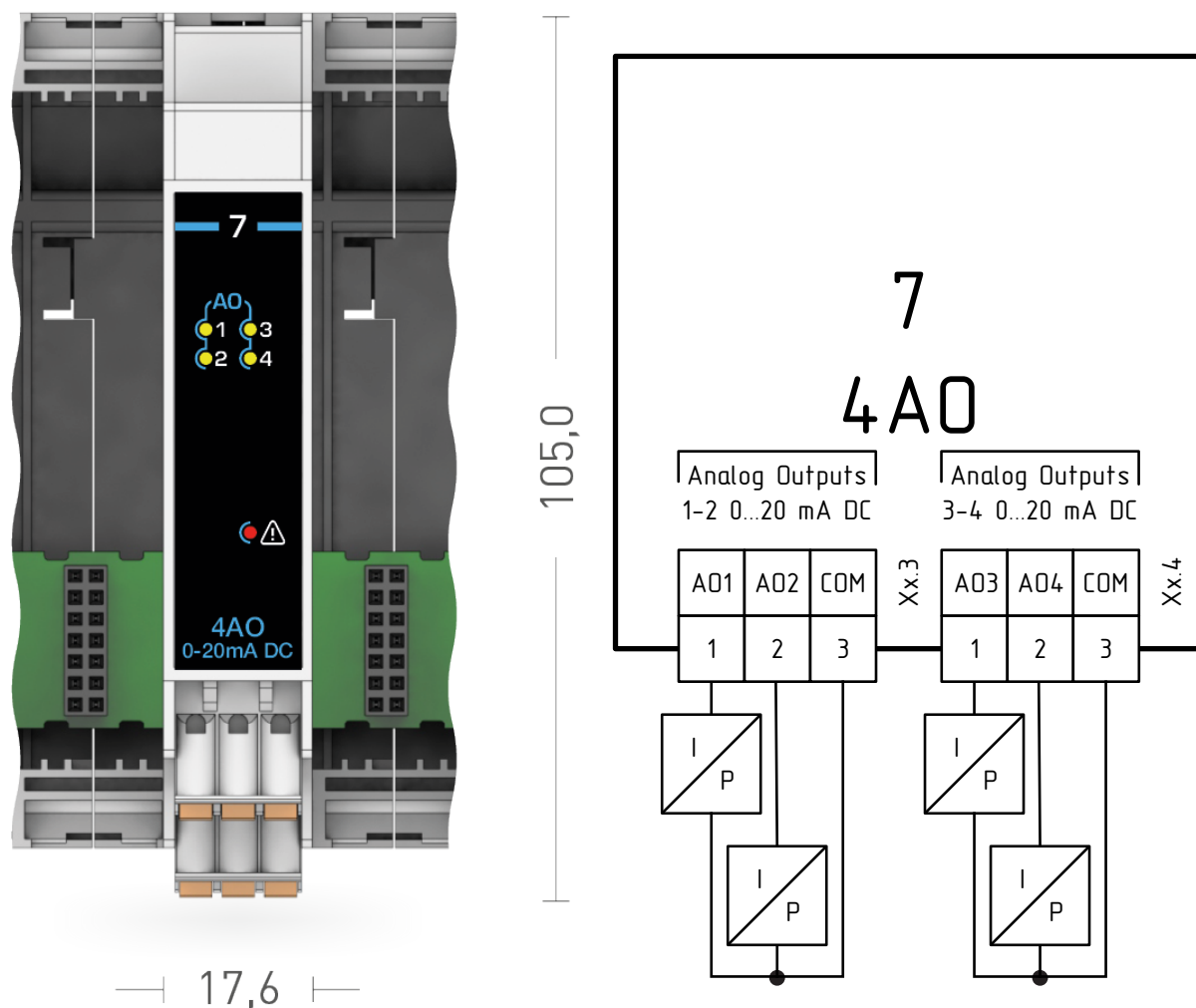
Рисунок 1.13 – Внешний вид и схема подключения модуля расширения MCU-7-4AO
